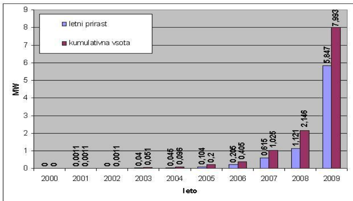
Slika 32: Rast fotovoltaike 2000–2009.
