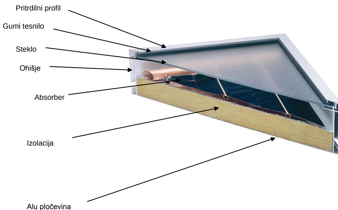
Slika 16: Sprejemnik sončne energije - prerez Vir: Programi za dimenzioniranje solarnega sistema IMP Klimat, MOP
