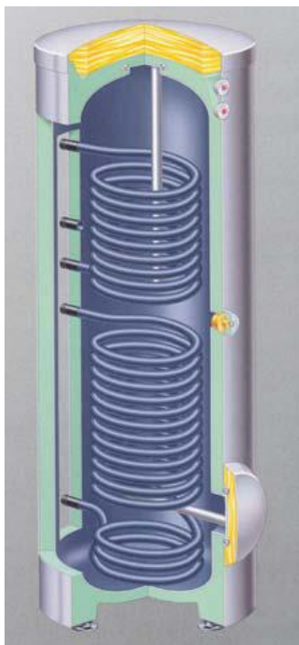
Slika 22: Hranilnik toplote.
